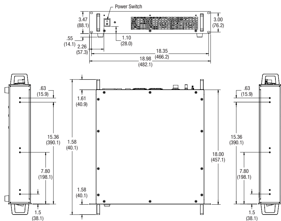
Utility Module Dimensions
